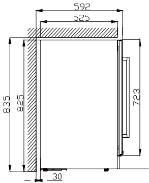
安裝側視圖
