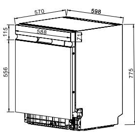
※ 中式廚櫃(高度800mm)
