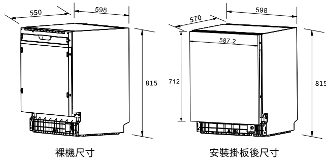
裸機尺寸
